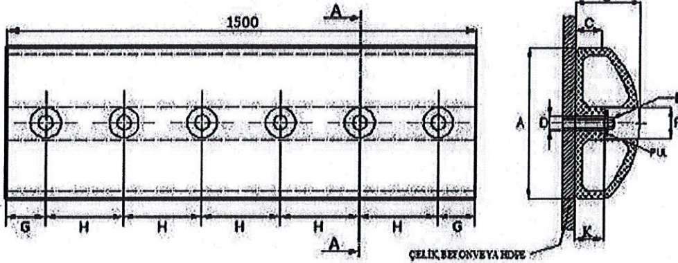
B TİPİ USTURMAÇA ÖLÇÜLERİ
